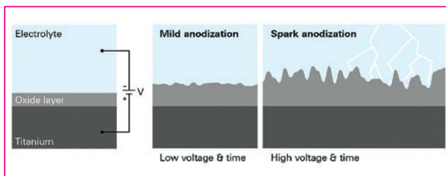
Für die Anodisierung wird Titan in eine Elektrolytflüssigkeit getaucht. Die Dauer und das Spannungsniveau bestimmen die Topografie der Oxidschicht.
